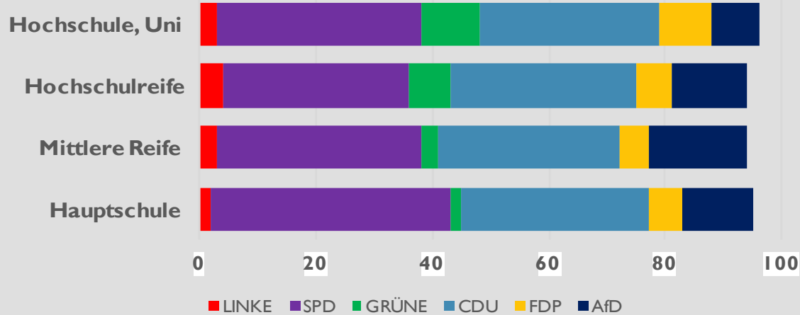
RP LTWI 6: Wahlverhalten nach Bildungsgrad
