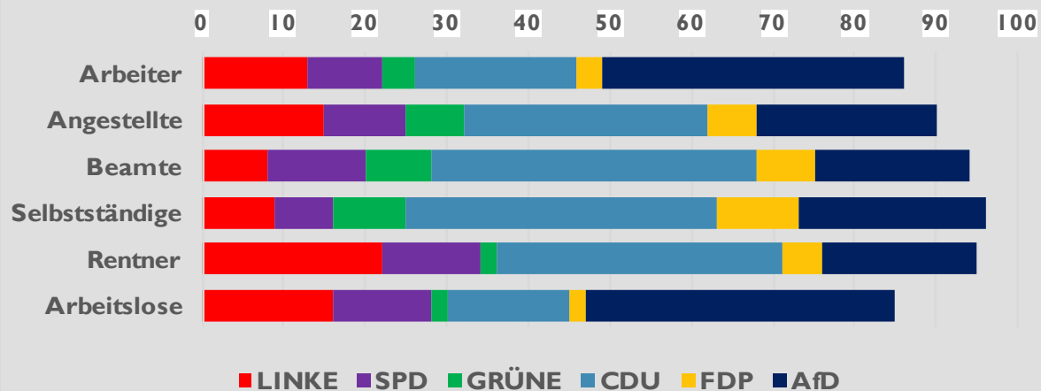
ST LTWI 6: Wahlverhalten nach Beruf/Tätigkeit
