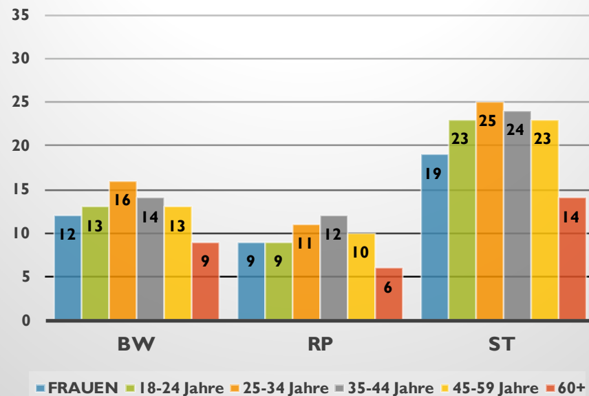
LTWI 16: AfD-Stimmenanteile unter Frauen
