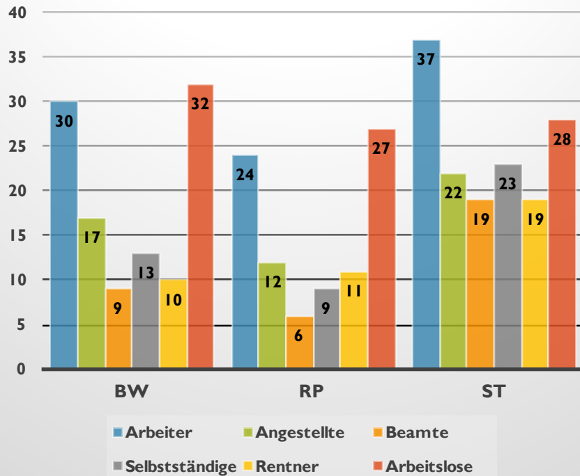
LTWI 6: AfD-Stimmenanteile nach Beruf/Tätigkeit
