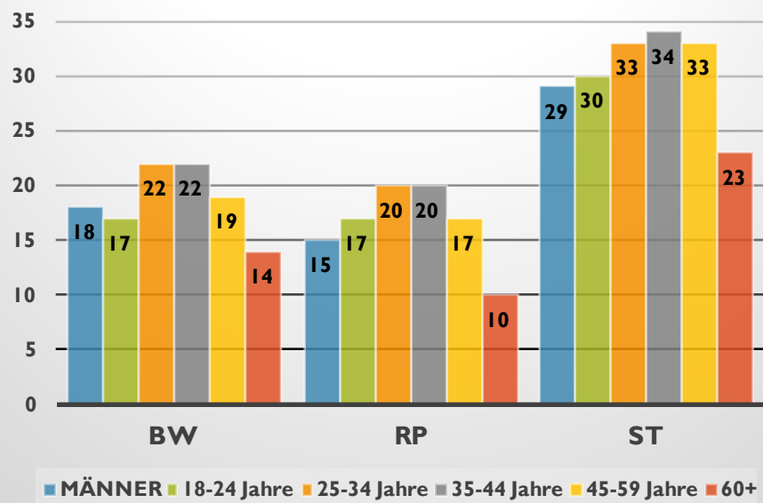
LTWI 16: AfD-Stimmenanteile unter Männern
