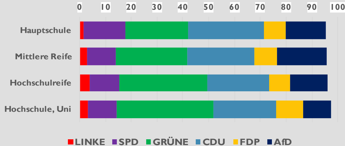
BW LTWI 6: Wahlverhalten nach Bildungsgrad
