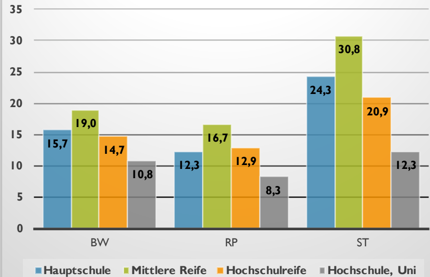
LTWI 6: AfD-Stimmenanteile nach formalem Bildungsgrad
