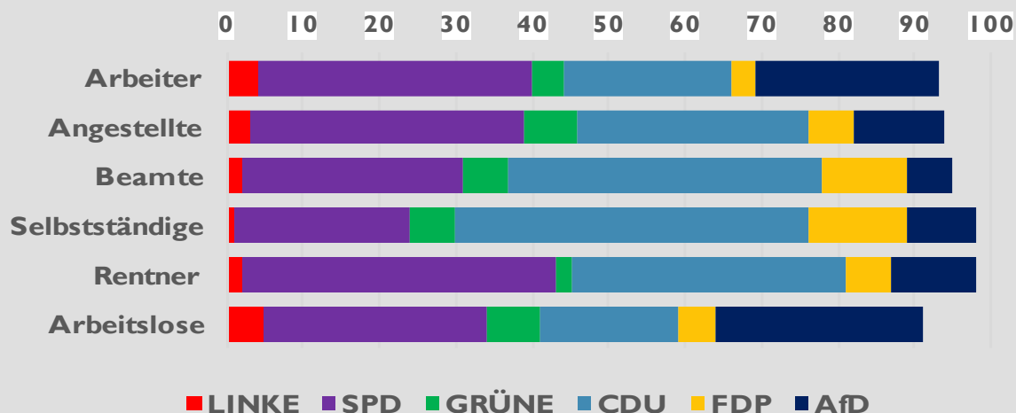
RP LTWI 6: Wahlverhalten nach Beruf/Tätigkeit
