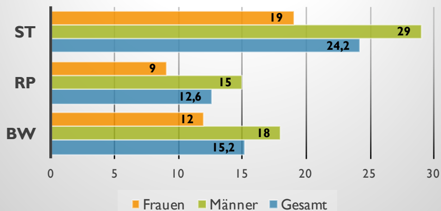
LTWI 16: AfD-Stimmenanteile nach Geschlecht
