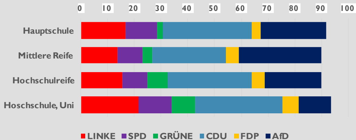
ST LTWI 6: Wahlverhalten nach Bildungsgrad
