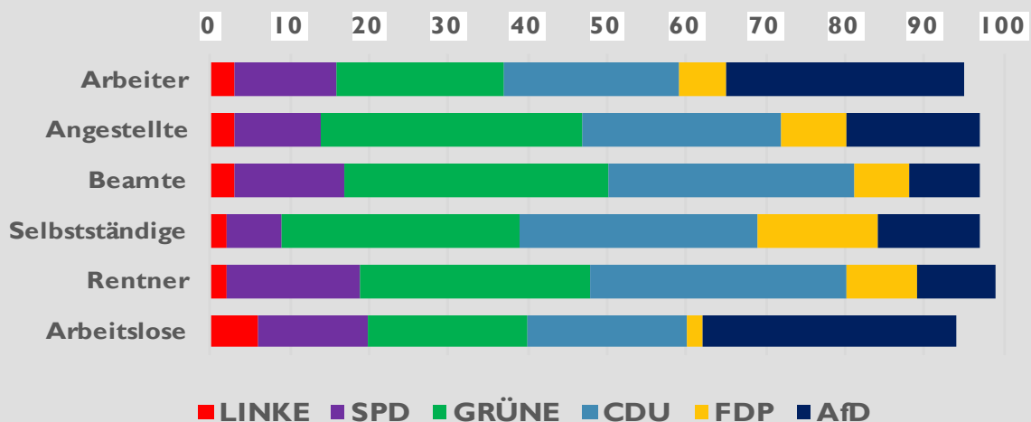
BW LTWI 6: Wahlverhalten nach Beruf/Tätigkeit
