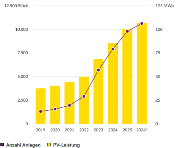
So viel Photovoltaik-Leistung ist in Oldenburg installiert In Megawatt-Peak (MWp), *Stand Juli 2026
