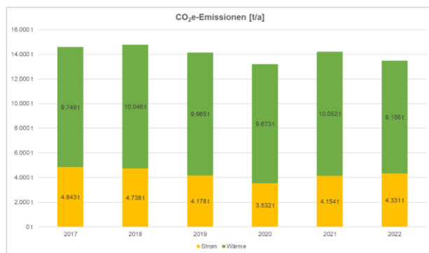
Abbildung 12: Treibhausgasemissionen der kommunalen Liegenschaften 2017 bis 2022 8
